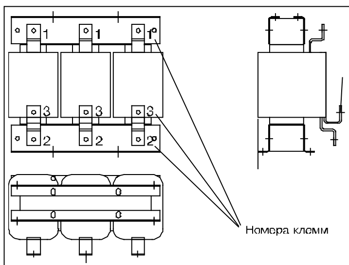
Рисунок 5-5. Входные дроссели
