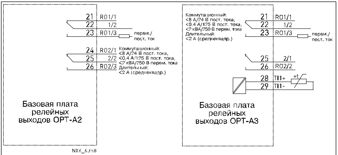
Рисунок 8-5. Принципиальная схема подсоединения базовых плат релейных выходов (OPT-A2/OPT-A3)
